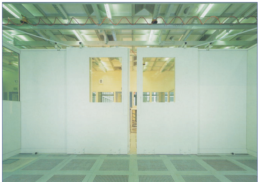
Metalltrennwand mit Bleieinlage (Strahlenschutzwand)
